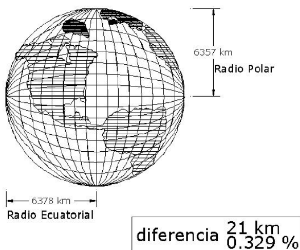
Figura : Esfericidad terrestre y su relación con el radio polar y el ecuatorial
