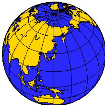
Figura : Proyección Ortográfica
