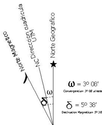
Figura : Convergencia de Meridianos
